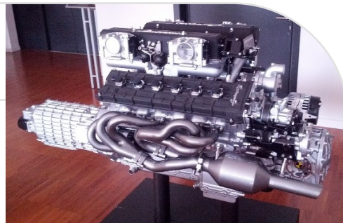
Museo Lamborghini (BO), motore 12 cilindri - Inarcassa 2016
