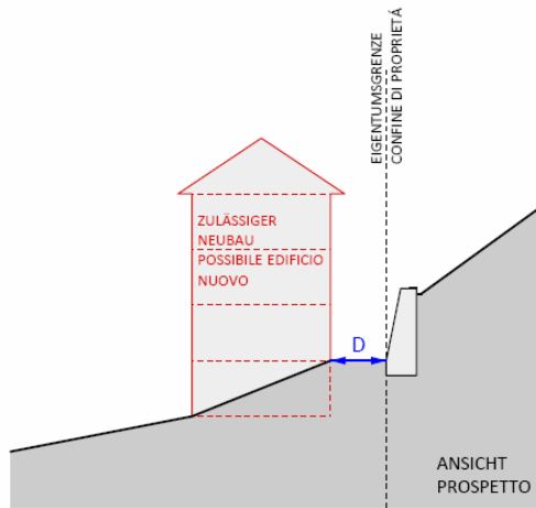
1.LÖSUNG/ SOLUZIONE 3m \leq D
